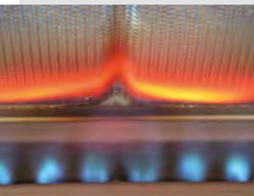
Brennereinheit mit Infrarotgitter
