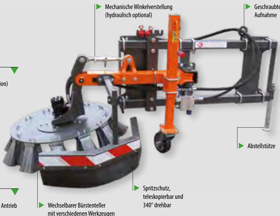
Bürstenteller 80 cm Durchmesser mit Zöpfen (Option)
