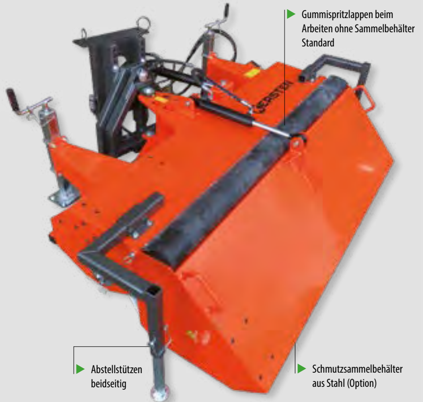
Mechanischer oder hydraulischer Antrieb möglich
