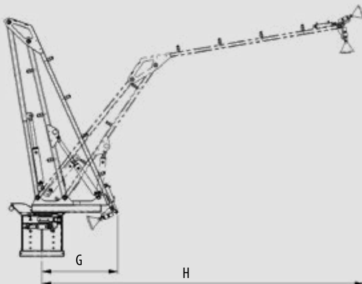
Vorderansicht
