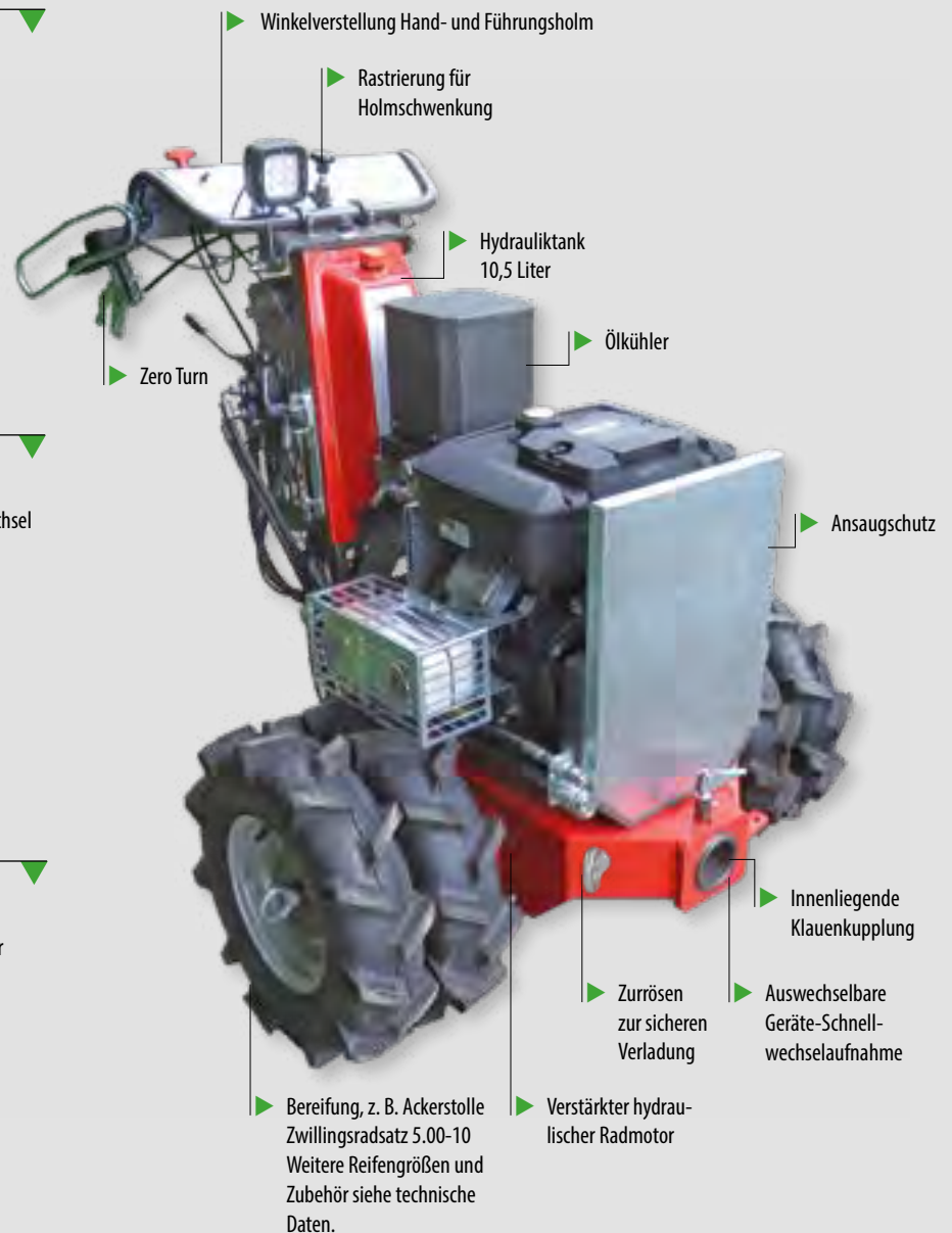
Stark dimensionierter Antriebsstrang
